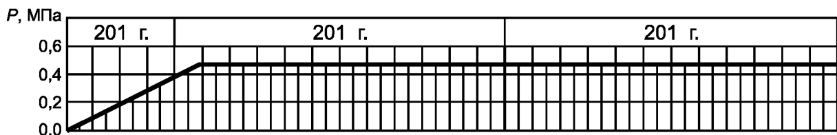
Рисунок Г.3 — График давления на основание фундамента
