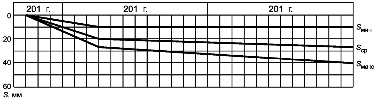
Рисунок Г.4 — График развития перемещений
