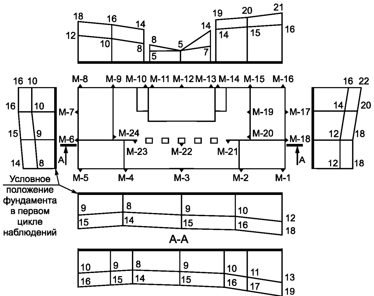
Рисунок Г.1 — Схема фундамента и основания
